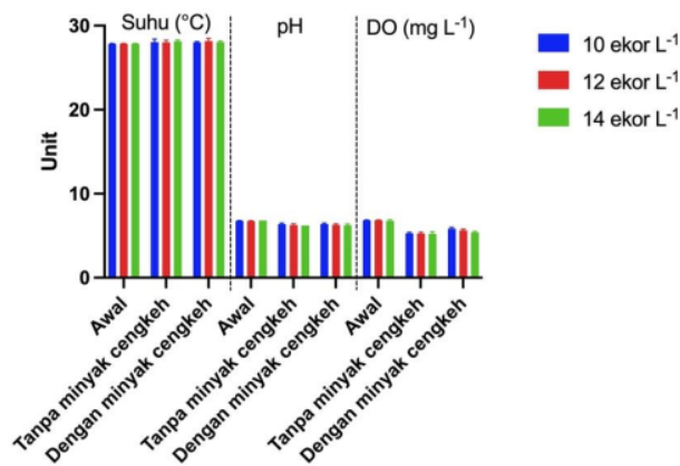
Gambar 2. Kualitas air (pH, oksigen terlarut, dan suhu) sebelum dan sesudah transportasi ikan tambakan dengan dan tanpa menggunakan minyak cengkeh
